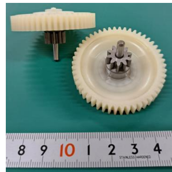
〈電動パーキングブレーキ構成部品〉 特徴:インサートモールド品
